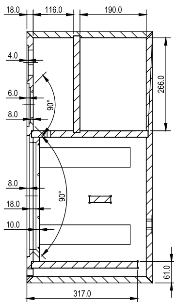
SECTION A-A SCALE 1 : 7
